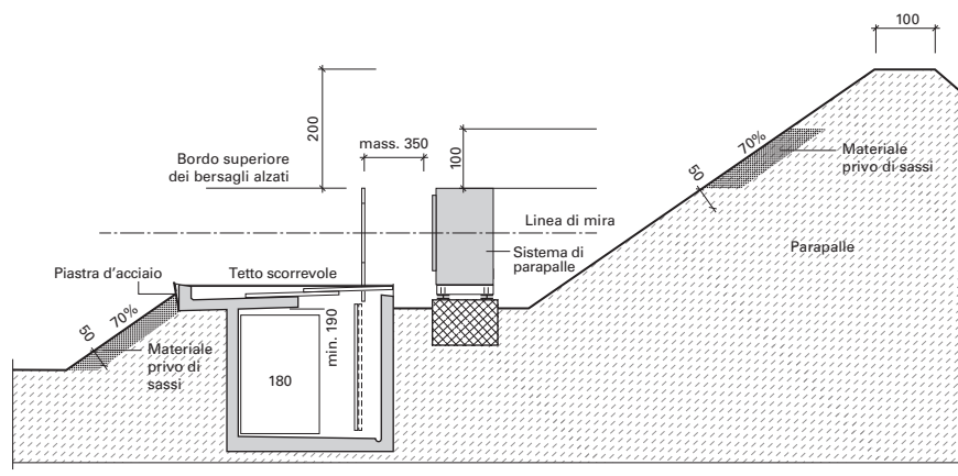
Fig. 42: Parapalle con materiale di riempimento
