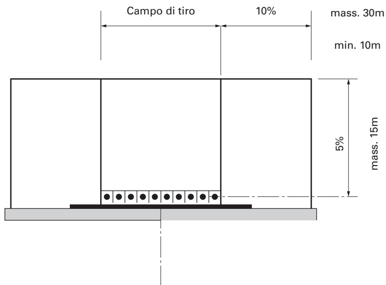
Fig. 8 Veduta (secondo regl sull'alta tensione)
