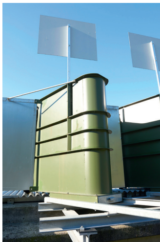
Fig. 52: Vista posteriore del sistema di parapalle, variante MaRep con cassetto
