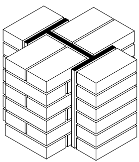
Detail Stützenkonstruktion
