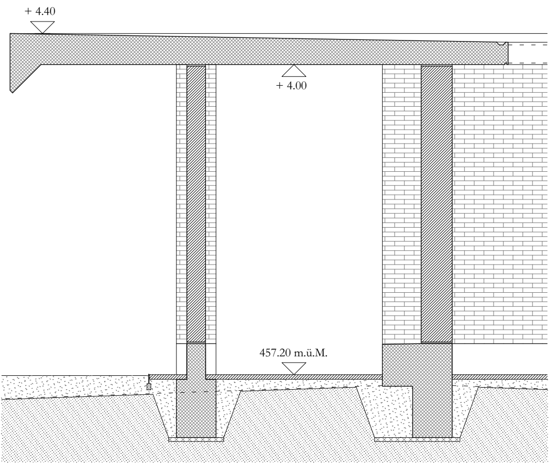
Detailschnitt 1 : 50
