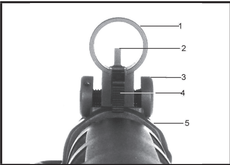
Fig. 9: Bloc-guidon
