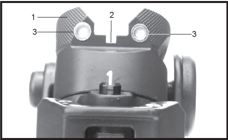
Fig. 8: Hausse « 1 »
