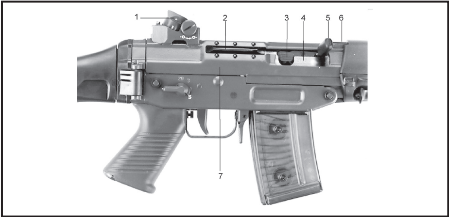
Fig. 3: Boîte de culasse
