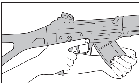
Fig. 69: Introduire un magasin
