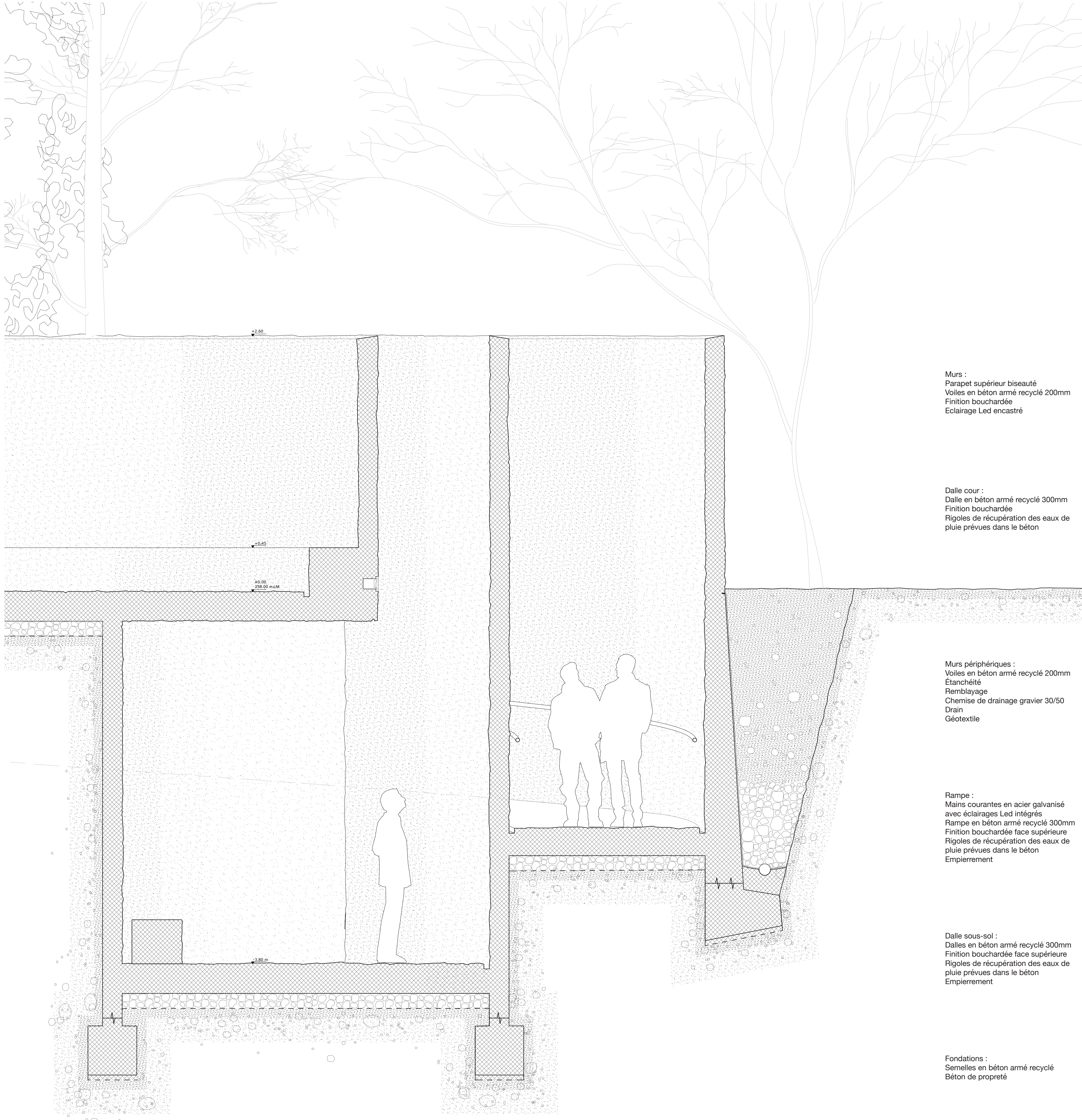
Coupe détail 1:20
