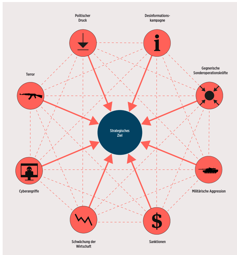
Abbildung 3: Bedrohung
