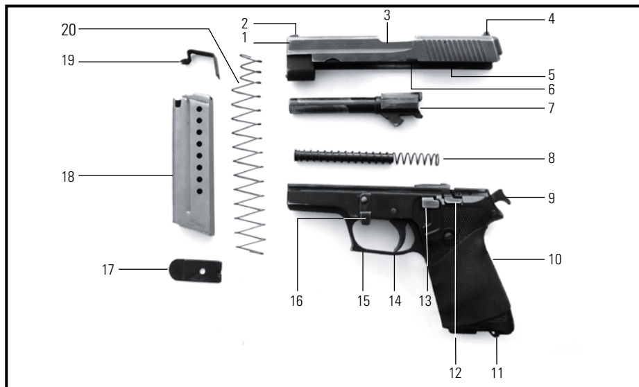
Abbildung 2: Die Bestandteile der Pistole 75
