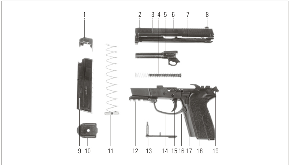
Abbildung 7: Die Bestandteile der Pistole 03
